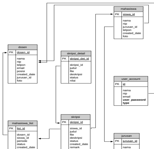
Gambar 4. Logical Record Structure Aplikasi Manajemen Skripsi
