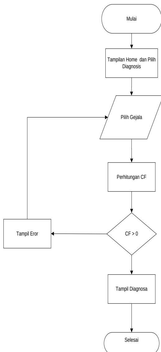
Gambar 4. Rancangan Algoritma
