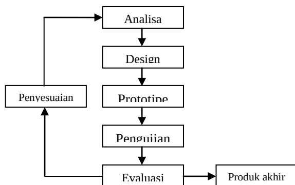
Gambar 3. Tahapan penelitian
