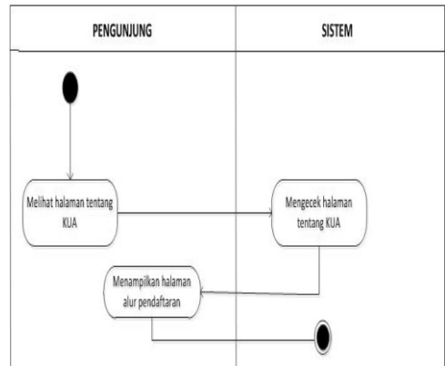
Gambar 9. Activity Diagram Pengunjung melihat alur pendaftaran nikah
