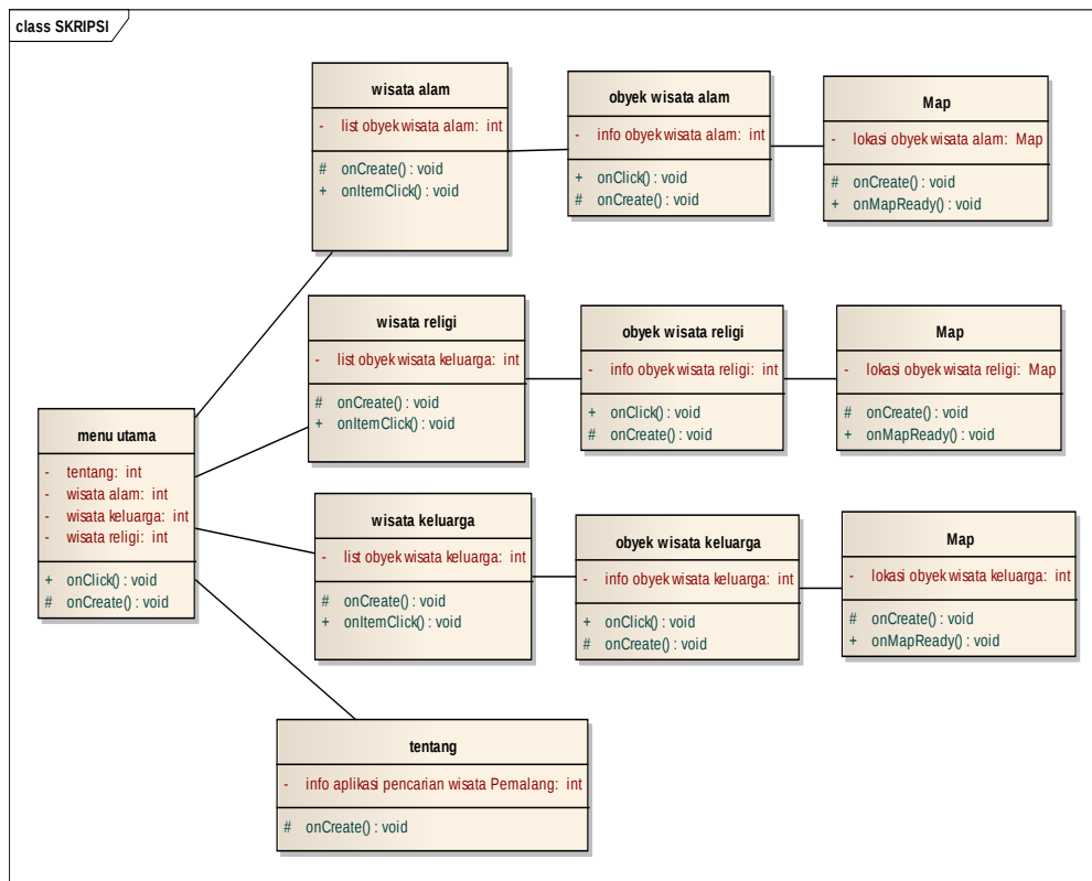
Gambar 1 Diagram class pencarian wisata Pemalang
