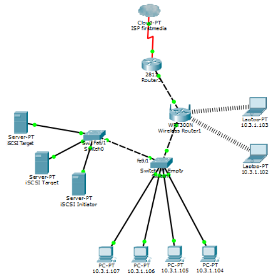
Gambar 4. Skema menggunakan Packet Tracer
