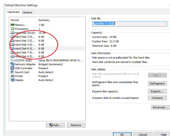
Gambar 12. Harddisk SCSI 5 telah dihapus
