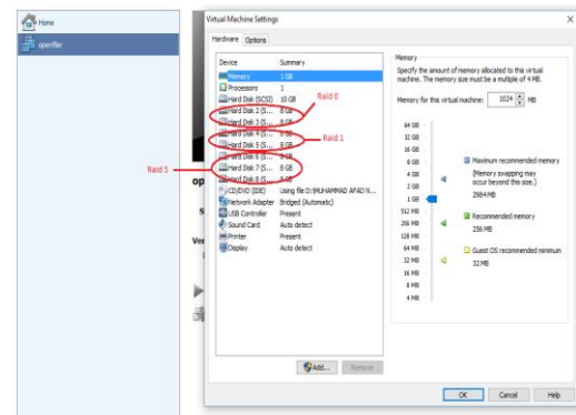
Gambar 8. Harddisk virtual untuk RAID
