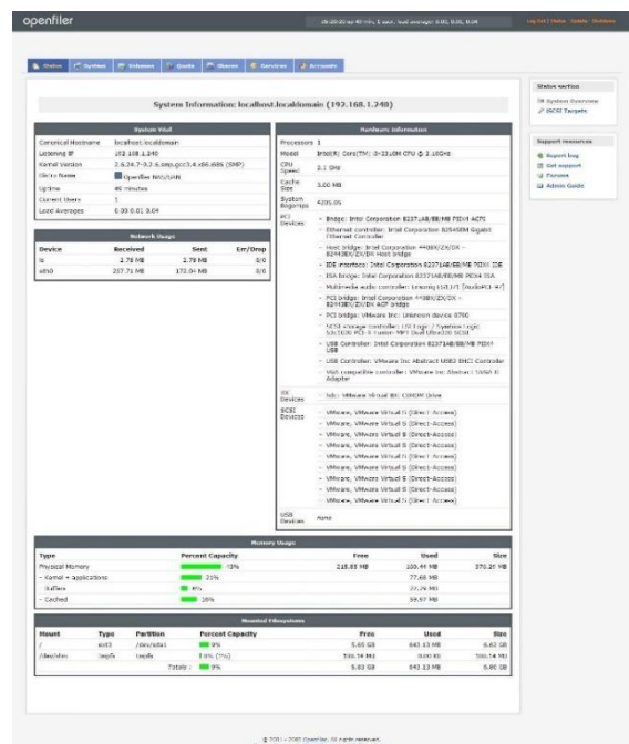
Gambar 5. Konfigurasi Openfiler
