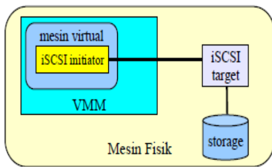
Gambar 3. Penerapan iSCSI
