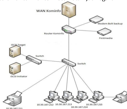
Gambar 2. Topologi Usulan
