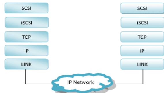
Gambar 1. Letak iSCSI
