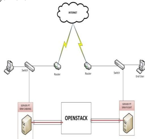
Gambar 6. Topologi usulan
