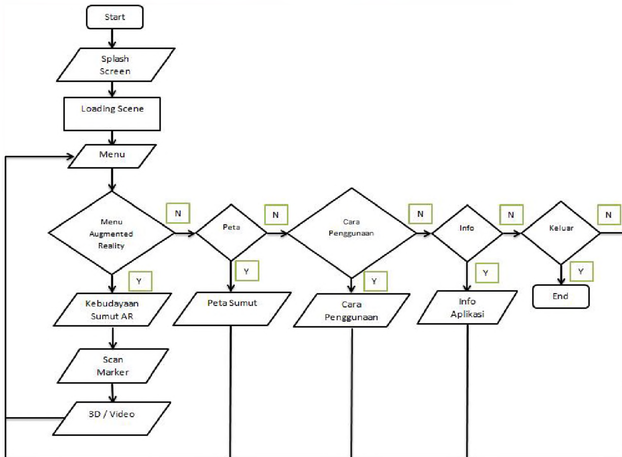
Gambar 1. Flowchart Navigasi Pengenalan Kebudayaan Sumatra Utara
