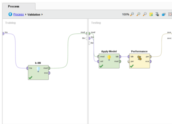
Gambar. 4. Implementasi Algoritma KNN
