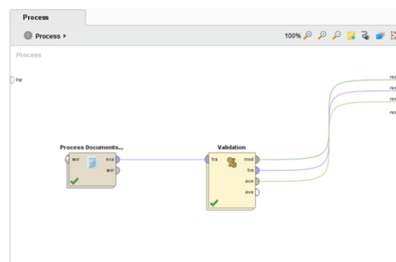
Gambar. 2. Implementasi Process Data dan Validation pada Algoritma Naive Bayes
