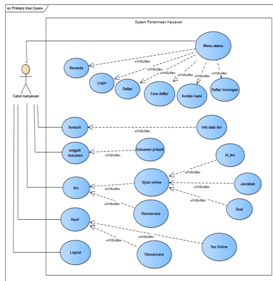
Gambar 1. Use case calon karyawan Tabel 1. Deskripsi use case calon karyawan
