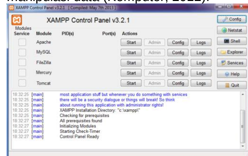
Gambar 2. XAMPP Version 1.8.2
