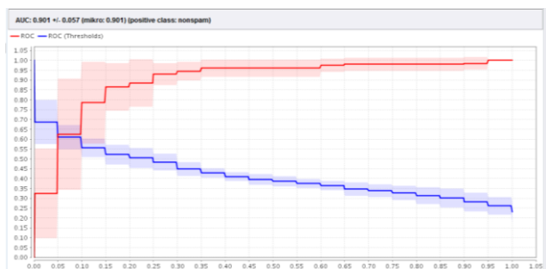
Gambar 8. Kurva ROC dengan metode Support Vector Machine
