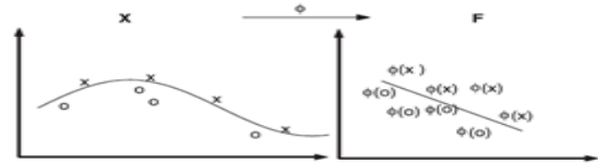
Gambar 1. Kernel map mengubah problem yang tidak linier menjadi linier dalam space baru
