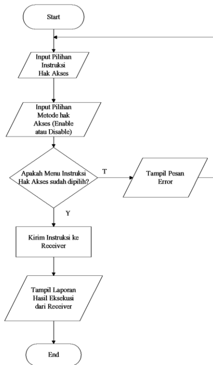
Gambar 12 Proses Pengiriman Instruksi dari Sender ke Receiver
