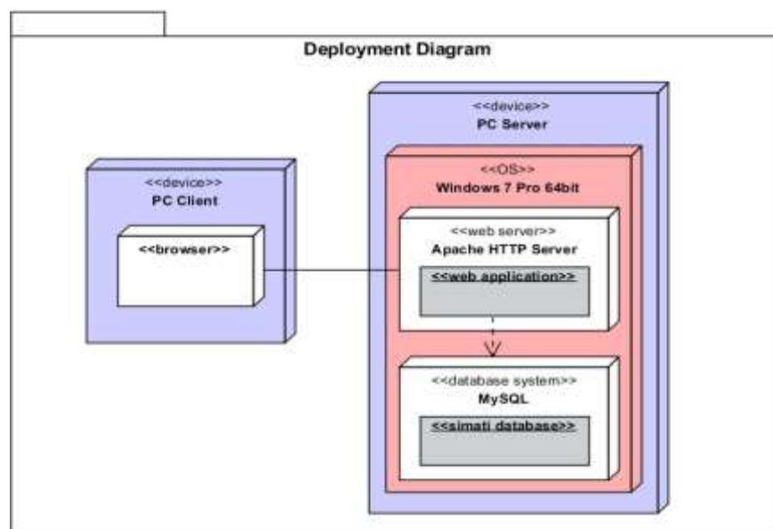
Gambar IV.20 Deployment Diagram Sistem Informasi Penjualan PT Hasta Prima Industri
