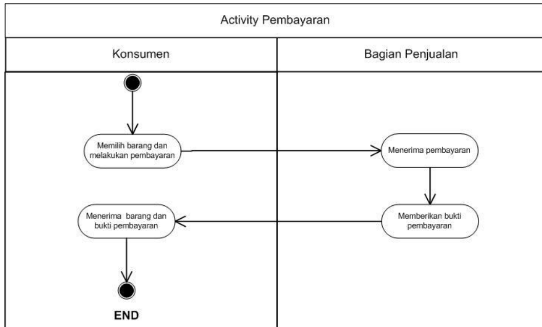
Gambar III.4. Activity Diagram Pembayaran Sistem Berjalan
