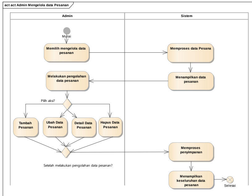
Gambar 4. Activity Diagram Mengelola Data Pemesanan
