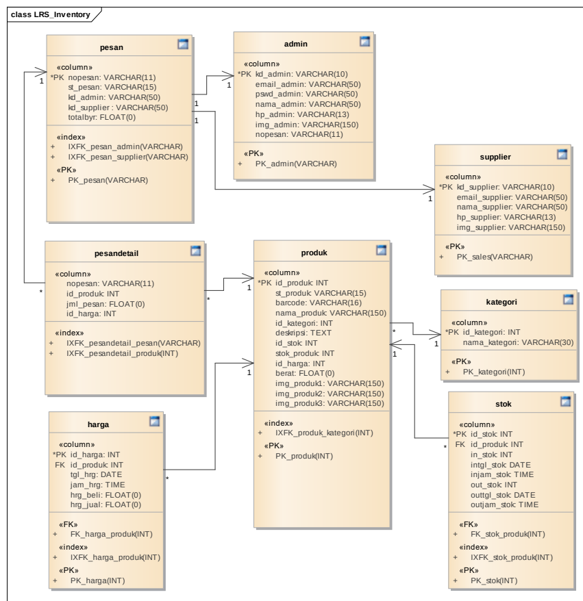
Gambar 2. Logical Record Structure (LRS) aplikasi Sistem informasi inventory
