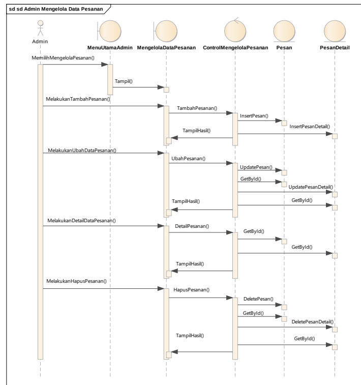
Gambar 5. sequence Diagram Mengelola Data Pemesanan
