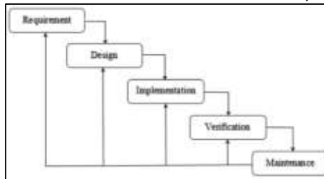
Gambar 1. Pemodelan Waterfall
