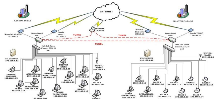
Gbr. 2 Skema Jaringan Usulan
