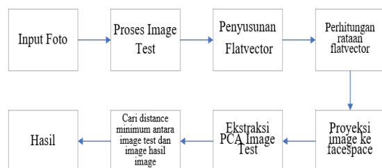
Sumber: Hasil Penelitian Gambar 1. Proses pengenalan Wajah
