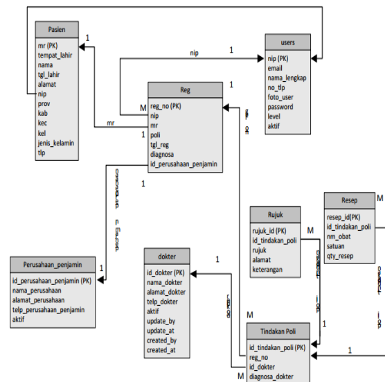
Gambar 1. Rancangan Database dengan LRS
