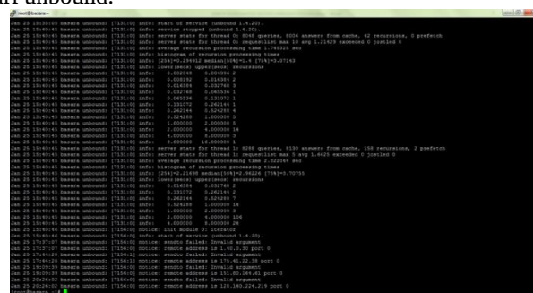
Gambar 19. Sample log dari unbound yang berjalan
