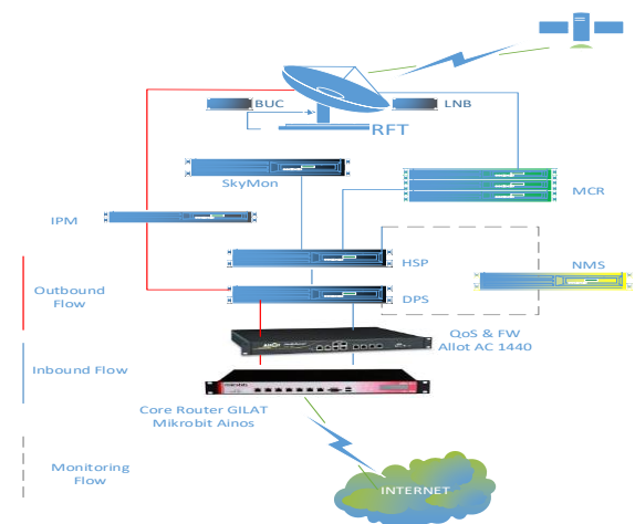
Gambar 2. Arsitektur Jaringan VSAT GILAT PT. indo Pratama Teleglobal
